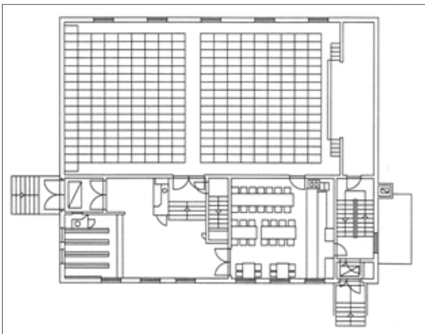
План 1 этажа Дома рабочих в Лаhti. Финляндия. 1965. Архив городского музея г. Лаhti
